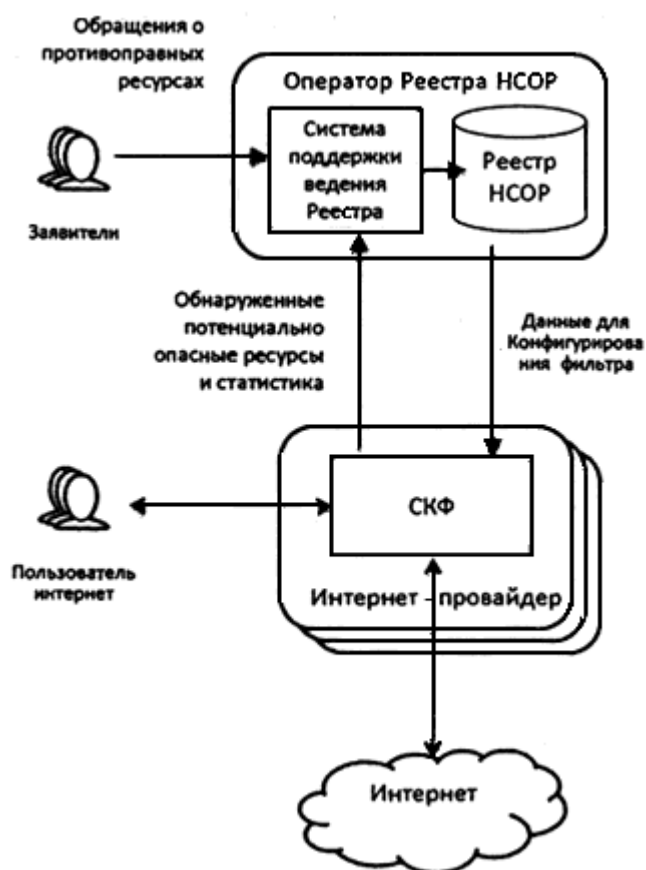
Рис. 6. Принцип контроля доступа через Реестр NSOP
