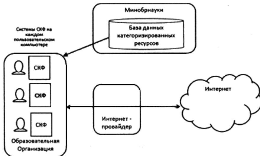
Рис.3. Схема работы контент-фильтрации при размещении в ОО
